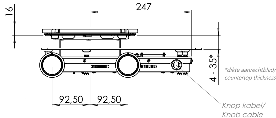
Vooraanzicht / Front view
