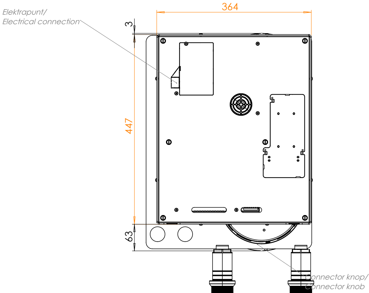
Onderaanzicht / Bottom view
