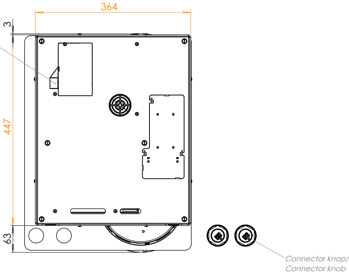
Onderaanzicht / Bottom view
