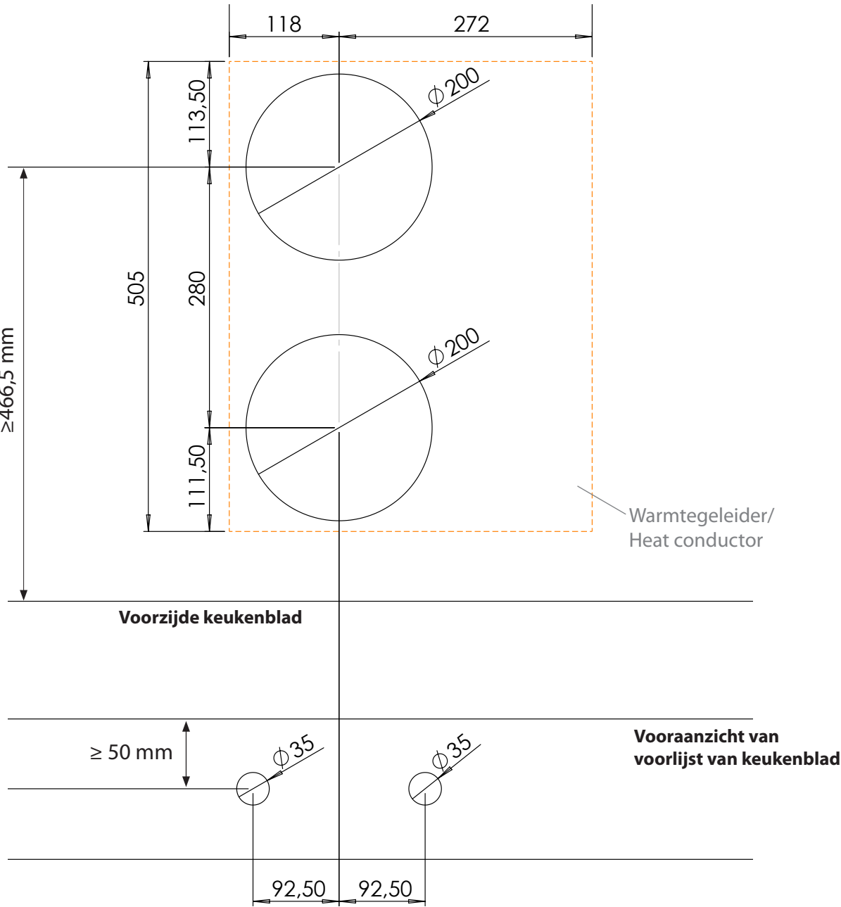
Gatenpatroon DXF bestand
