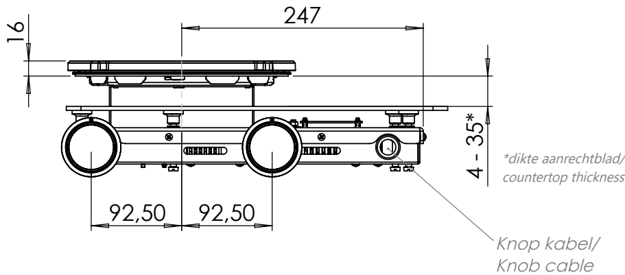
Vooraanzicht / Front view
