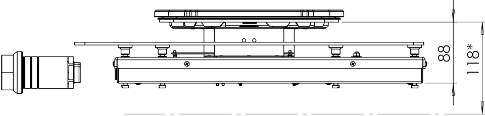
Zijaanzicht / Side view
