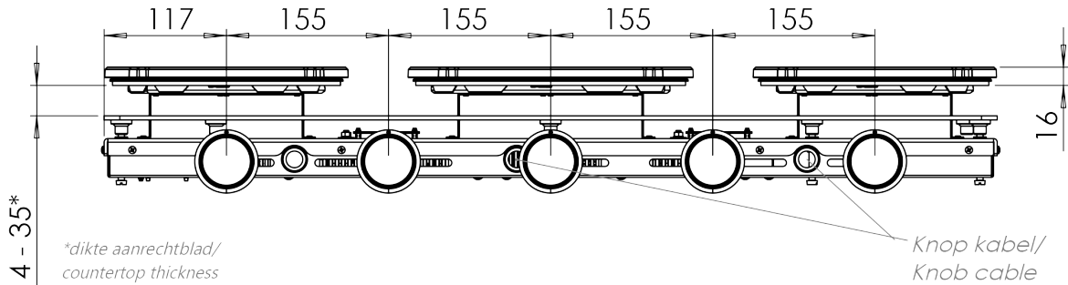
Vooraanzicht / Front view
