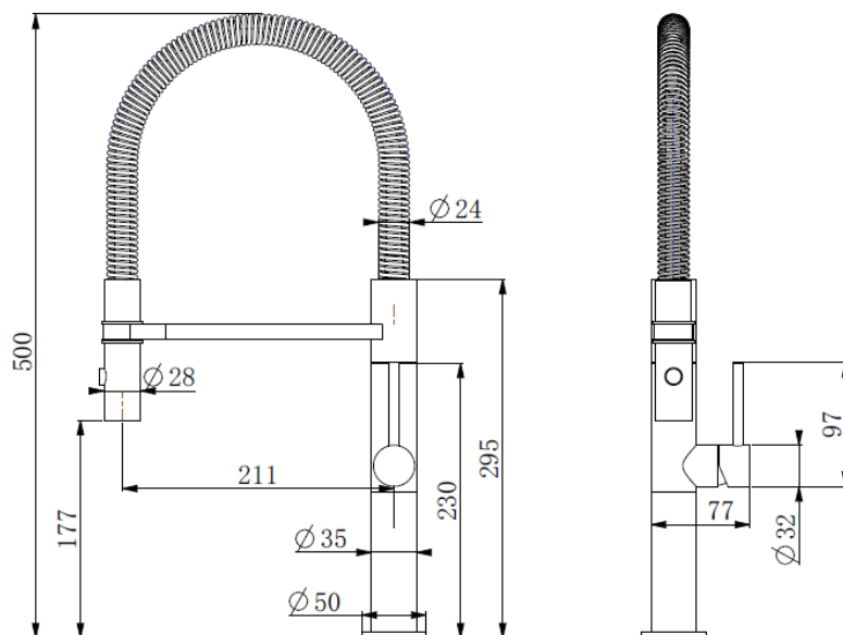
Dimensions
